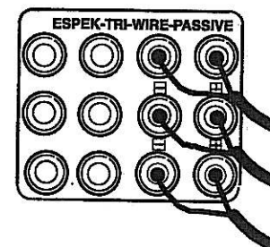
パッシブ方式： (トライワイヤー配線)
