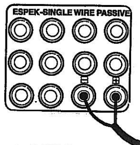
パッシブ方式： (シングルワイヤー配線)
