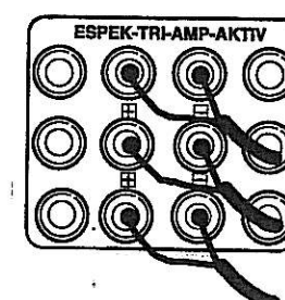
トライアンプ・アクティブ方式： (3台のパワーアンプを使用したマルチアンプ駆動)
